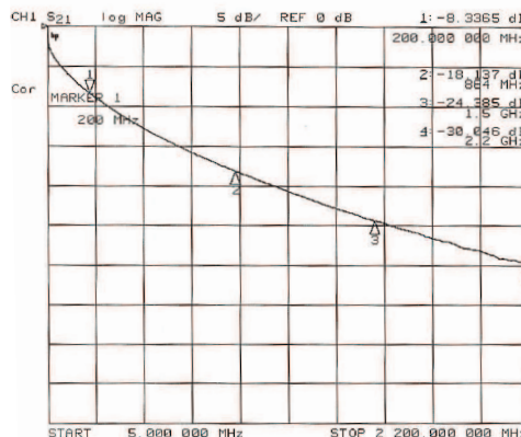
Rysunek 3: Tłumienność kabla NS113 TRI
