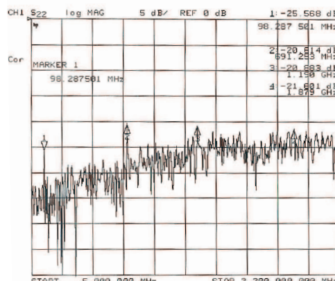
Rysunek 5: Tłumienność odbiciowa kabla NS113 TRI - port 2
